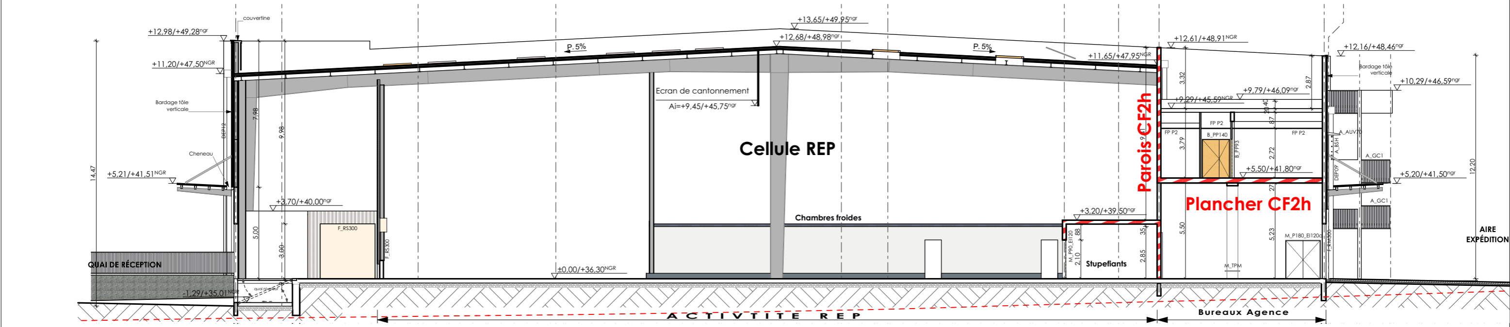
COUPE C
